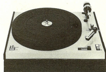
Philips Hi-Fi-stereopladespiller GA 317. I nederste højre hjørne ses pick-up-armens hæve- og sænkeanordning. Når pladen er færdigspillet, hæves armen automatisk.
