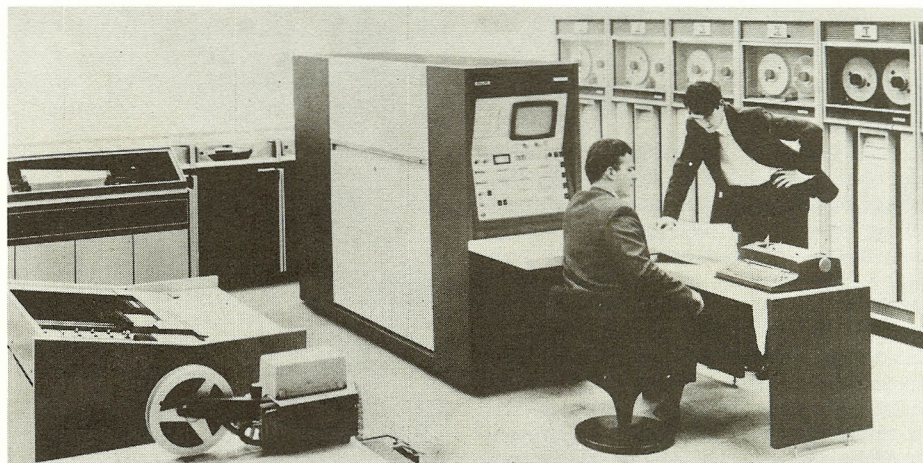
En foreløbig udgave af dataanlæg P-1100. Det er den ene af P-1000 seriens 3 modeller, som her er klar til afprøvning på Philips Computer. Industries i Apeldoorn.
