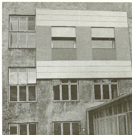
Prøveopsætning af glasemaileret facadeelement på Industrigården. Solafskærmningen er tænkt anvendt på vest- og sydvendte facader.
